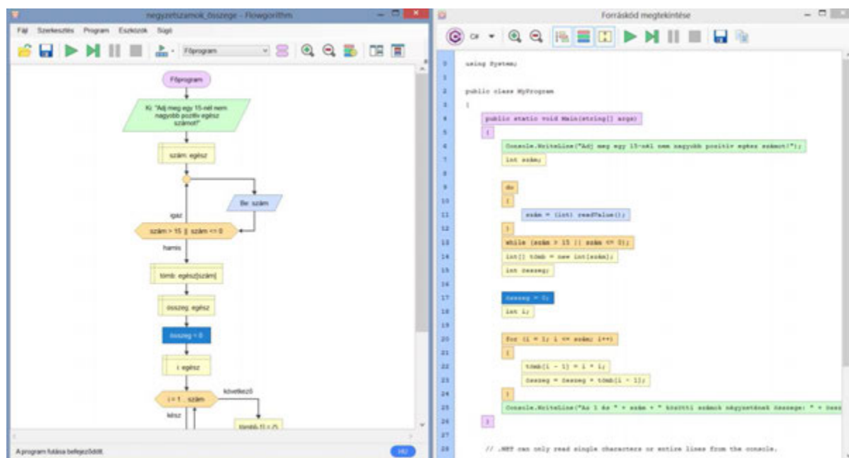
16. ábra: Az algoritmus és a hozzá tartozó forráskód
