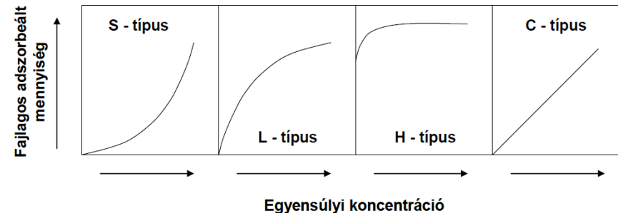
2.1. ábra: Híg oldatokra vonatkozó adszorpciós izoterma-típusok (Giles-féle izotermaosztályok)
